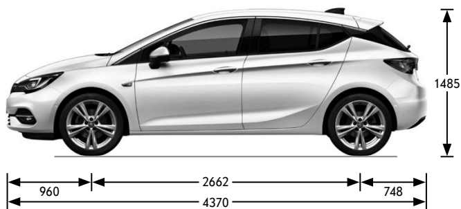
Astra 5-Türer Alle Maße in mm
