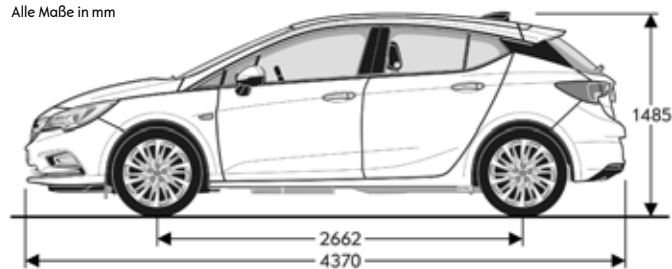
Astra 5-Türer Alle Maße in mm
