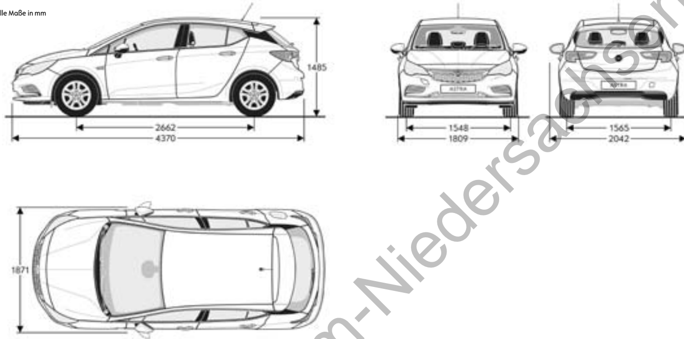
Breite mit eingeklappten Außenspiegeln 1871 mm
