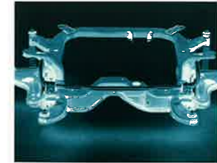
Der Fahrscmel mit 6 Entkopplungspunkten optimiert Fahrkomfort und Handling.
