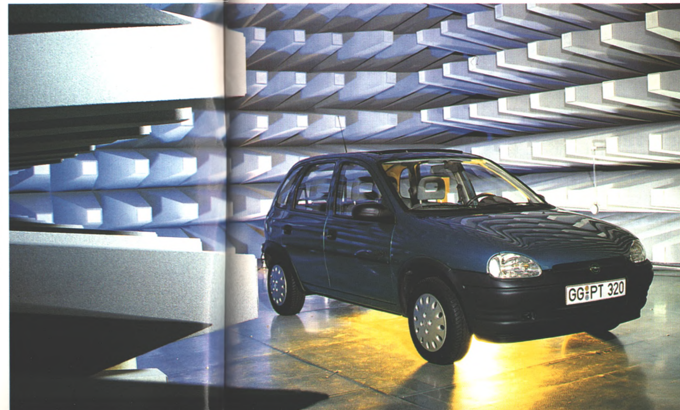
Als Problem für die empfindliche Elektronik im Auto können sich Strahlen von Hochspannungsleitungen, Rundfunkstationen usw. erweisen. In einem Labor zur Untersuchung elektromagnetischer Verträglichkeit simulieren Opel-Ingenieure auch extreme Belastungen. Seite 58.
